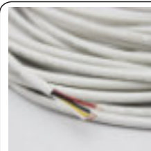
Przewód RGB okrągły 4-żyłowy 4x0,22 mm
